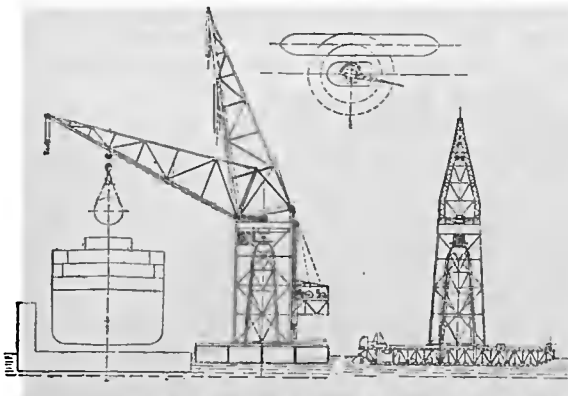
Плавучій кранъ въ Гокоско.
